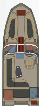
VENTURA 220 WS p. 24
