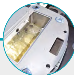
VIVIER EN ALUMINIUM ProFlo MD dans le module arrière incluant rebord anti-éclaboussures, trop-plein, lumière, recirculation intermittente et filtre protecteur sur la pompe de remplissage
