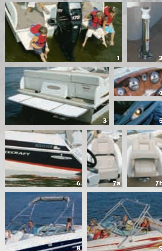
1 Plates-formes de baignade côtés conducteur et passager 2 Mât de remorquage (Vacanza seulement) 3 Plate-forme de baignade pleine largeur avec échelle d'embarquement (Ventura 190 L I/O seulement) 4 Instrumentation SmartCraft MD (Vacanza seulement) 5 Lumières d'accostage à halogène 6 Bande contrastée optionnelle (Vacanza seulement) 7 Siège capitaine avec coussin "bolster", glissières et plaque pivotante 8 Ensemble pour planche nautique en acier inoxydable (Vacanza) 9 Ensemble pour planche nautique en aluminium (Ventura 190 L et 190 LW)
