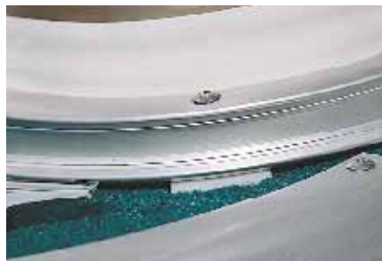
Rails surélevés Nos rails sont légèrement surélevés par rapport au pont pour permettre à l'eau accumulée sur le pont de mieux s'écouler.
