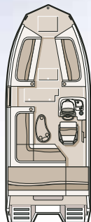
VACANZA 210 I/O (avec moteur 3.0 L)
